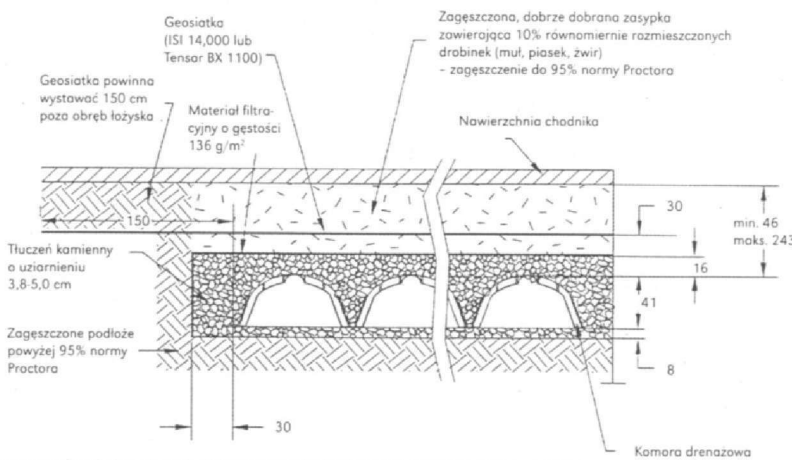
Przekrój poprzeczny przez system komór drenażowych. Uwaga: Zakład dwóch kolejnych rolek geosiatki wynosi 60 cm
