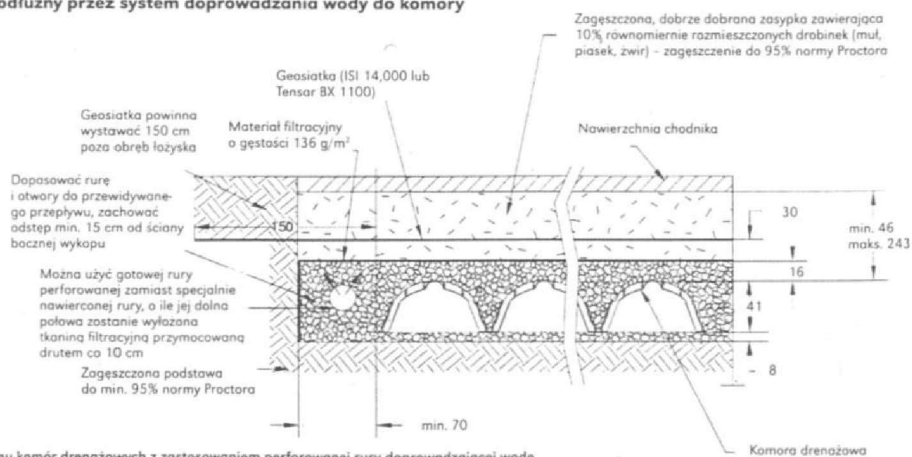
Przykład systemu komór drenażowych z zastosowaniem perforowanej rury doprowadzającej wodę
