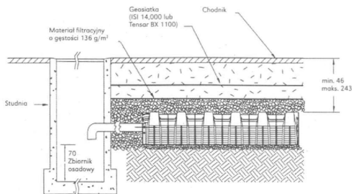
Przekrój podłużny przez system doprowadzania wody do komory
