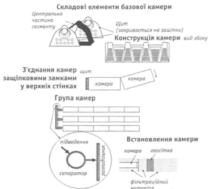
Рис. 6. Інфільтраційні камери INFILTRATOR
