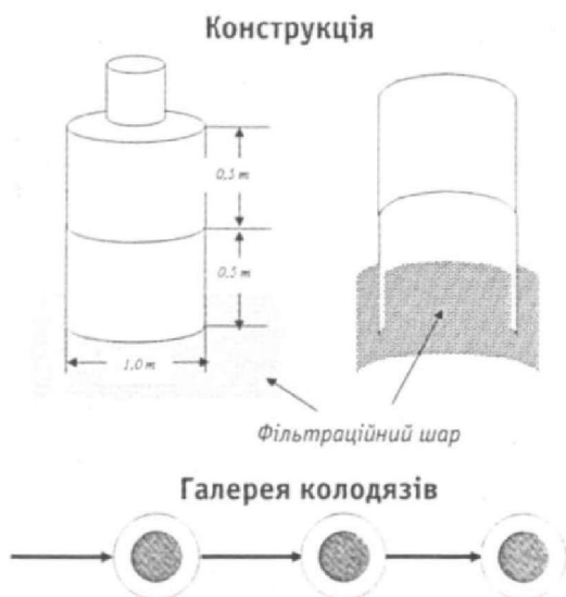
Рис. 5. Поглинальний колодязь AQUATRAIN
