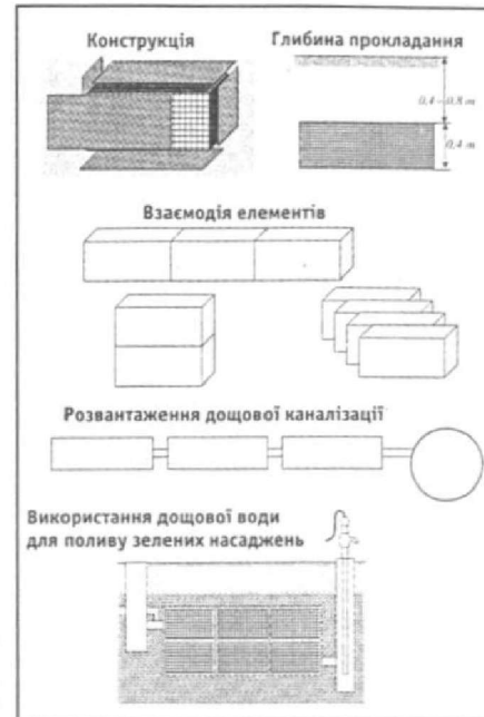
Рис. 3. Відведення дощових вод за допомогою лотків
