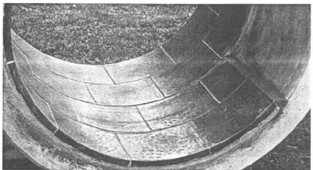
Rys. 9. Rura betonowa z wykładziną bazaltową. Wątpliwości wzbudza znaczna liczba fug oraz zastosowane wypełnienie – nie udało się uzyskać odpowiedzi na pytanie, jak się ono zachowa w warunkach podwyższonej agresywności środowiska
