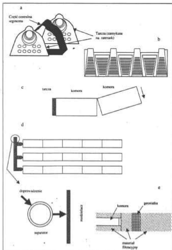
Rys. 3. Komory filtracyjne: a - zasada konstrukcji na przykładzie systemu INFILTRATOR, b - przekrój podłużny, c - zasada łączenia ze sobą komór, d - doprowadzenie wody do układu, e - zasada stosowania obsypki
