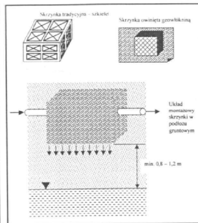
Rys. 5. Ogólny schemat skrzynki rozszczepiającej (na przykładzie konstrukcji firmy WAVIN)
